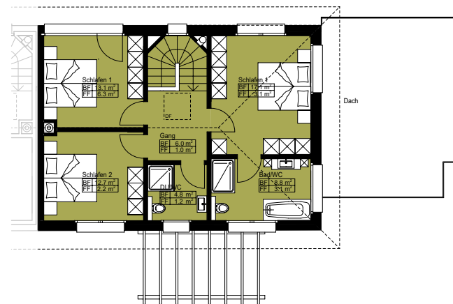
Obergeschoss 1:200
