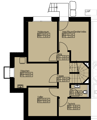
Kellergeschoss 1:200
