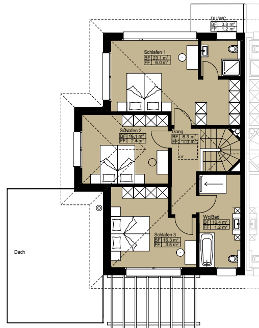
Obergeschoss 1:200
