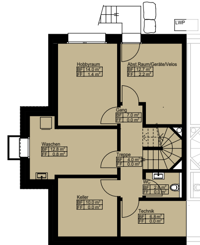
Kellergeschoss 1:200
