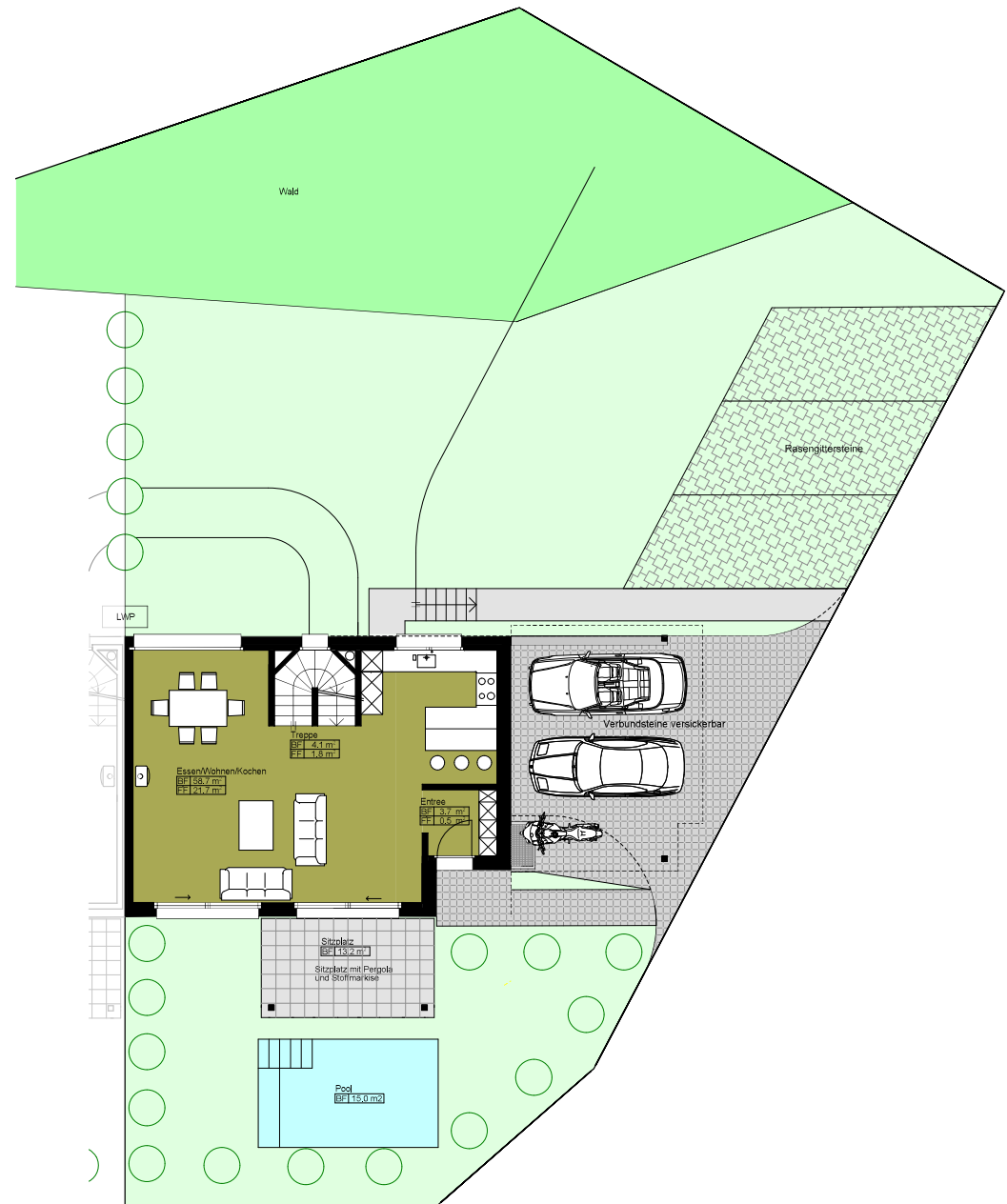
Erdgeschoss 1:200
