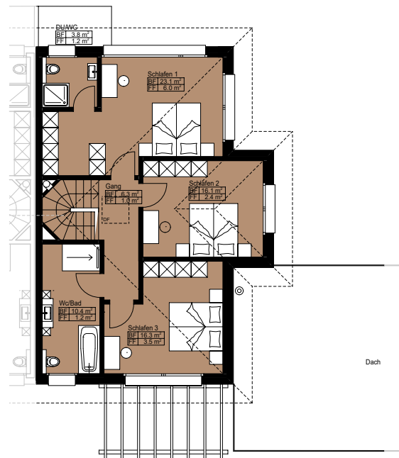
Obergeschoss 1:200
