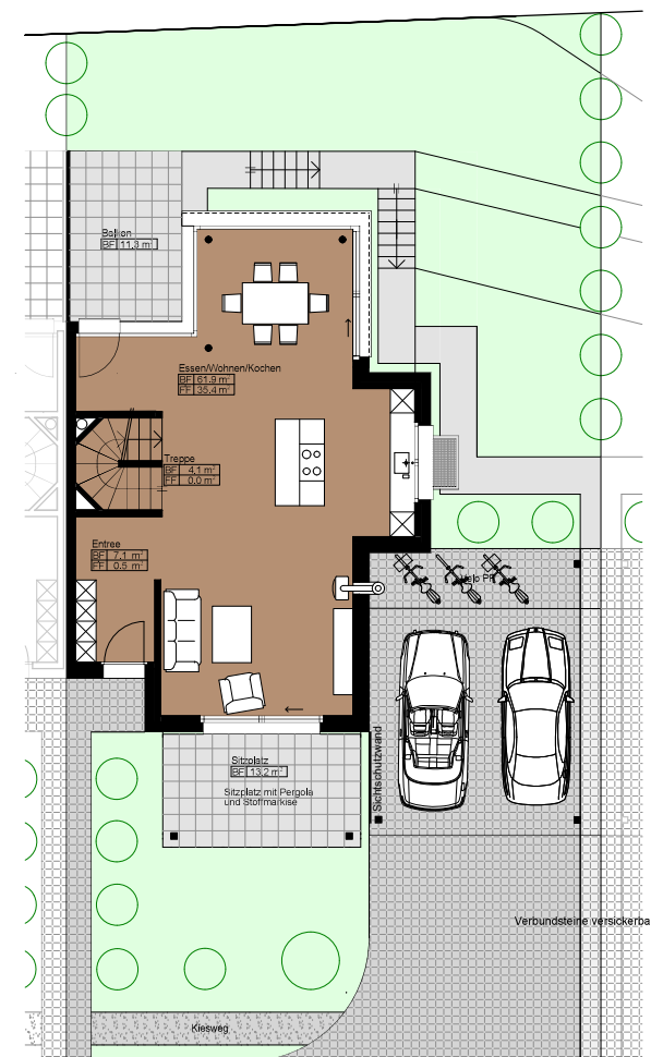
Erdgeschoss 1:200
